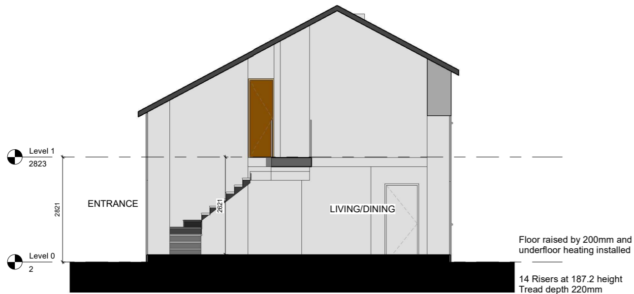
2 Section 2 1 : 50
